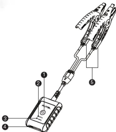
图 11-1 MaxiBAS BT506 电池诊断仪示意图
