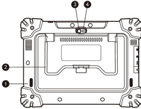
图 2-2 MaxiSys 平板电脑后视图
