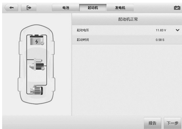
图 12-7 “起动机检测结果”界面示意图
