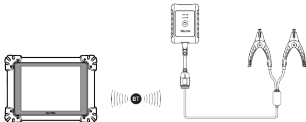
图 12-2 电池与平板建立通讯示意图
