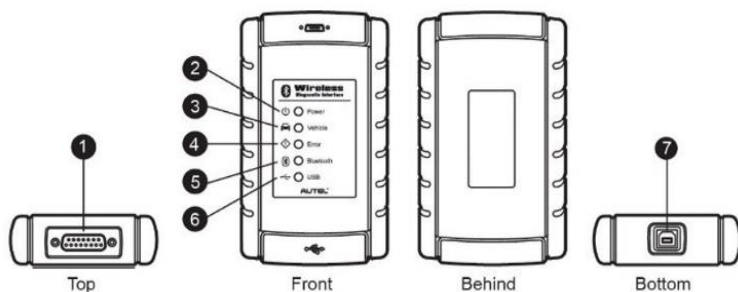
图 2-5 蓝牙诊断接口设备
