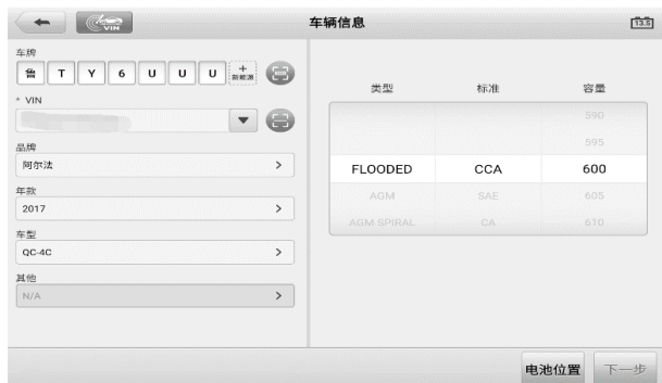
图 12-4 “电池检测”界面示图
