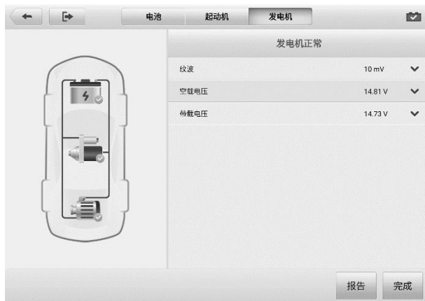
图 12-8 “发电机检测结果” 界面示意图
